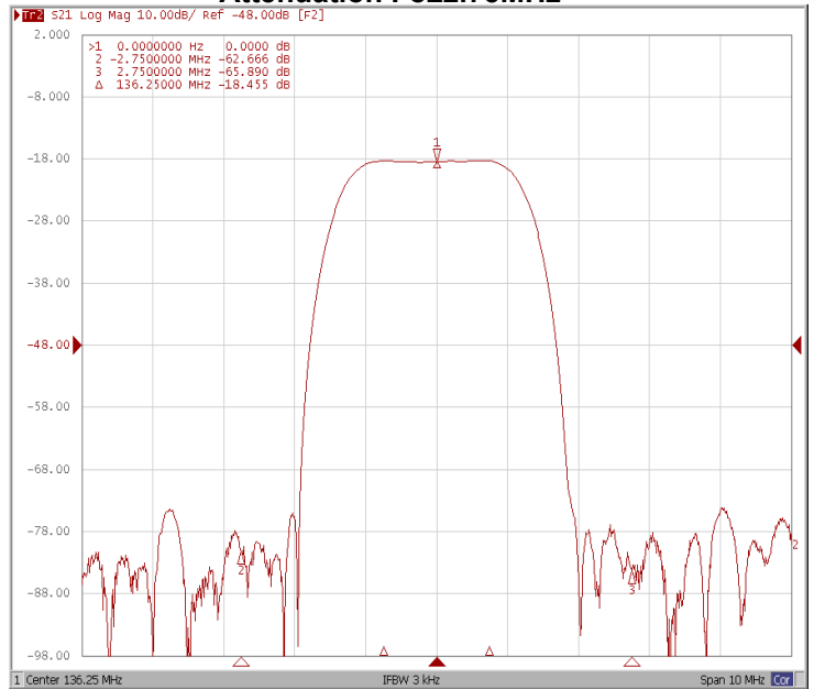
Attenuation Fo±2.75MHz
